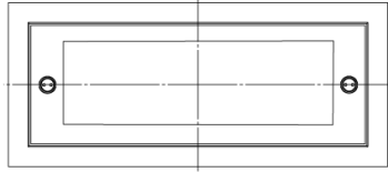
Dimensions d'encastrement 310
