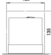
Dimensions d'encastrement 120
